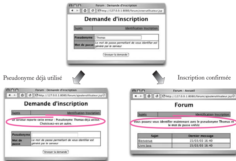
Figure 13-9 Résultat de l'inscription avec la page ajouterutilisateur.jsp
