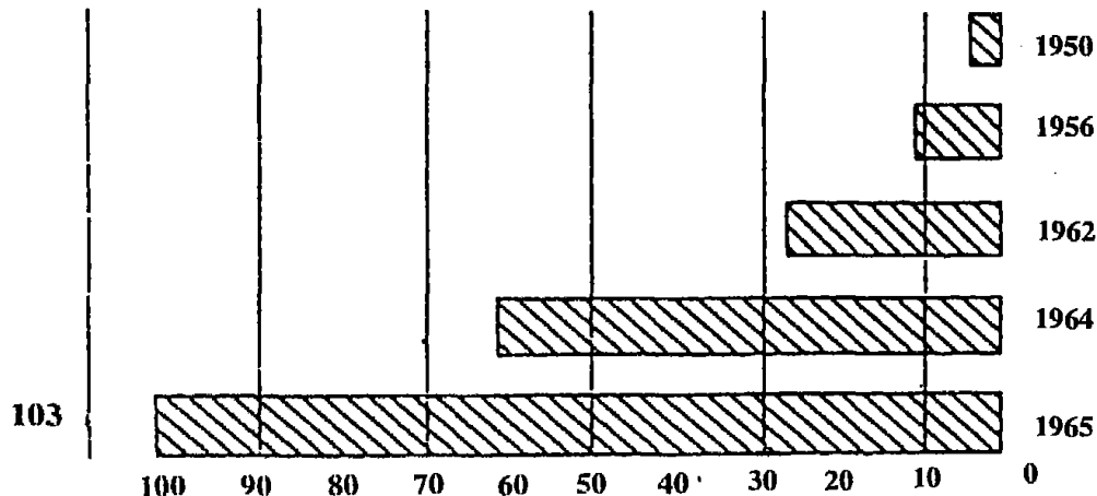
شكل (2): المدرج التكراري: ميزانيات (أوجه الصرف) للمكتبات العامة (مقدرة بملايين الدولارات)
