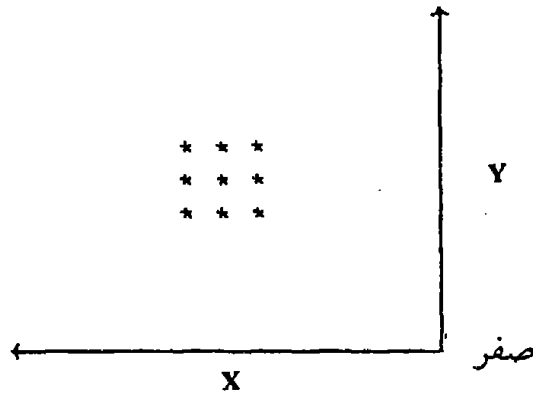
شكل (19): شكل انتشار يوضح عدم ارتباط بين المتغيرات (x) و (y)
