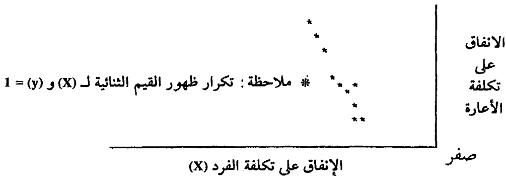
شكل (17): شكل انتشار يحتوي على نقط بيانات لـ 10 مكتبات، بالنسبة إلى متغيرين (x) و (y)
