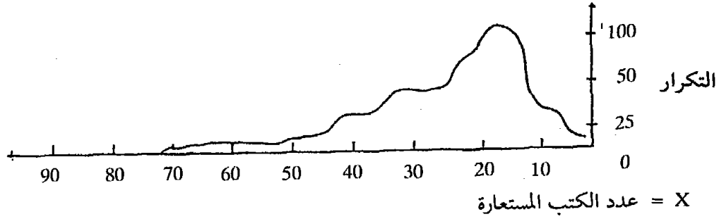
شكل (10): التوزيع التكراري النظري للمجتمع الكلي للمستفيدين من المكتبة، على ضوء العدد المتغير للكتب المستعارة
