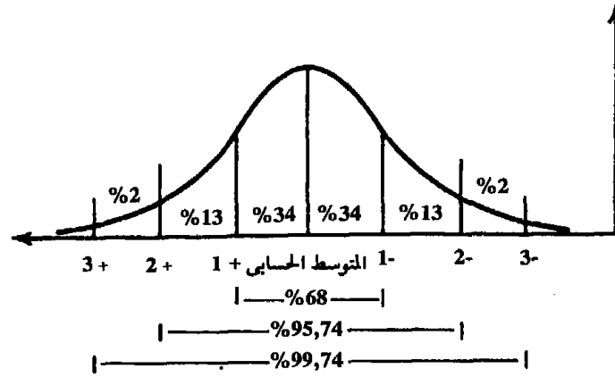
شكل (7) توزيع طبيعي يشير إلى مواقع الوحدات 1, 2, 3 للانحراف المعياري، لكل جانب من جانبي المتوسط الحسابي
