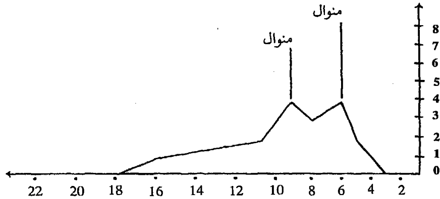
شكل (4): عرض مرتبات العاملين بالمضلع التكراري نموذج توزيع ثنائي
