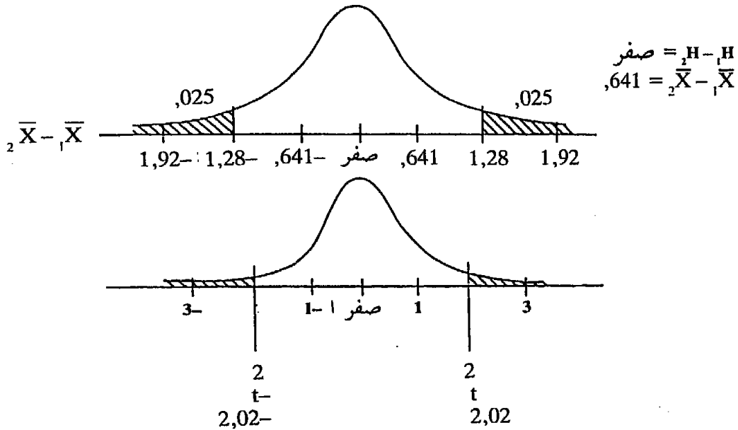
شكل (16): توزيع معانية إحصائية للفرق مابين المتوسطات الحسابية للعينة، مستنداً على حجم العينات: n_1 = 20 ، n_2 = 30 ، توزيع مطابق لـ t .
