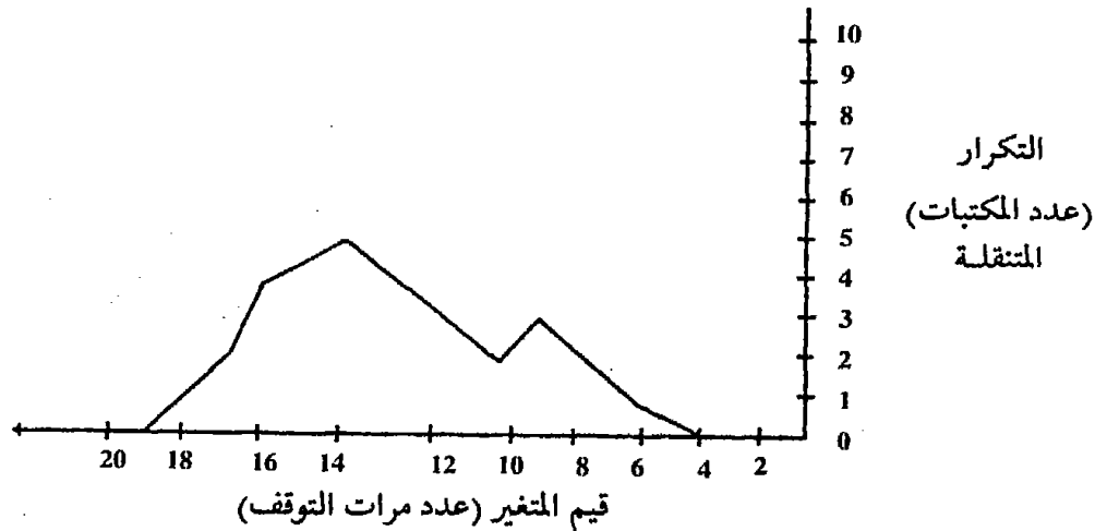
شكل (1): عرض مرات التوقف لـ 17 مقاطعة بالمضلع التكراري.
