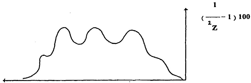
شكل (8): توزيع متعدد النماذج
