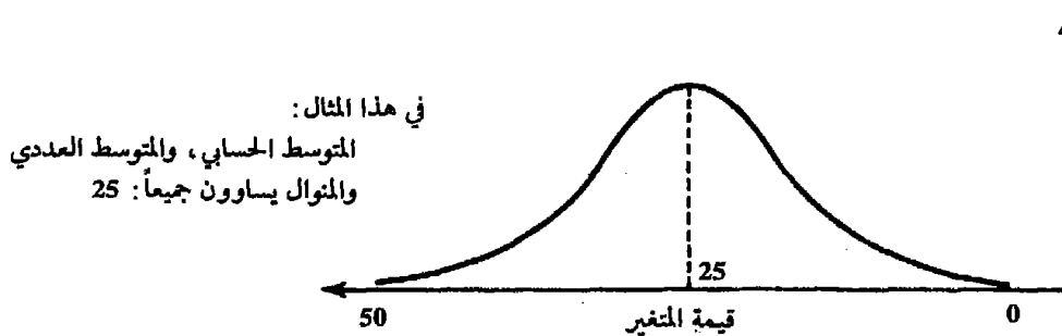
شكل (5): التوزيع الطبيعي ، مع المتوسط الحسابي لمجتمع دراسة يساوي 25.
