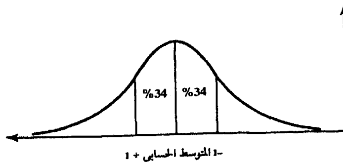
شكل (6) توزيع طبيعي ، يشير إلى وحدة انحراف معياري واحدة أسفل وأعلى المتوسط الحسابي .
