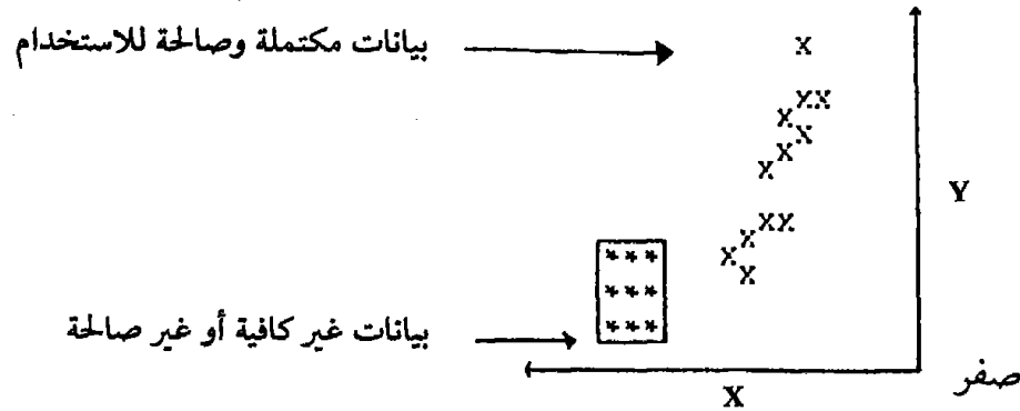
شكل (20): شكل انتشار، يوضح عينة غير ممثلة لمجتمع الدراسة ، مما ينتج عنها ، تقديرات واهية للارتباط بين المتغيرين (x) ، (y)
